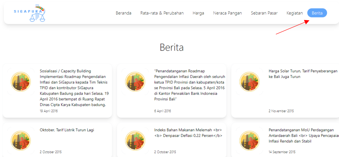
Gambar 8.9. Berita
