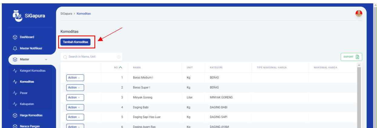
Gambar 3.18. Tambah Komoditas
