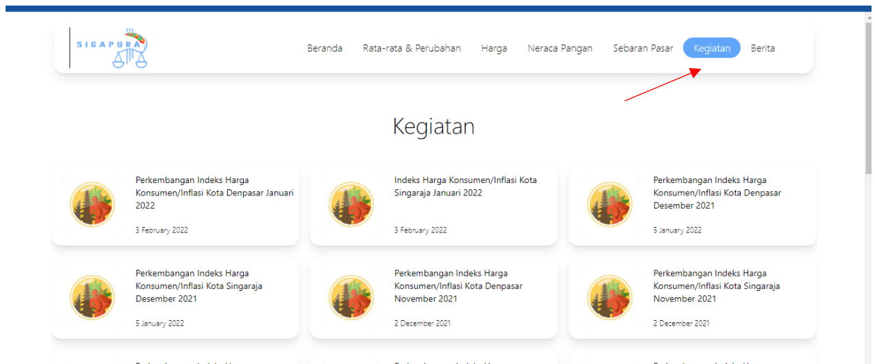
Gambar 8.8. Kegiatan
