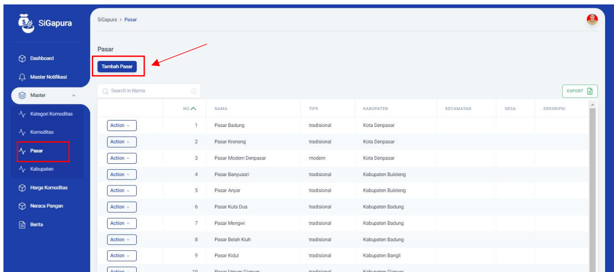
Gambar 3.26. Tambah Pasar
