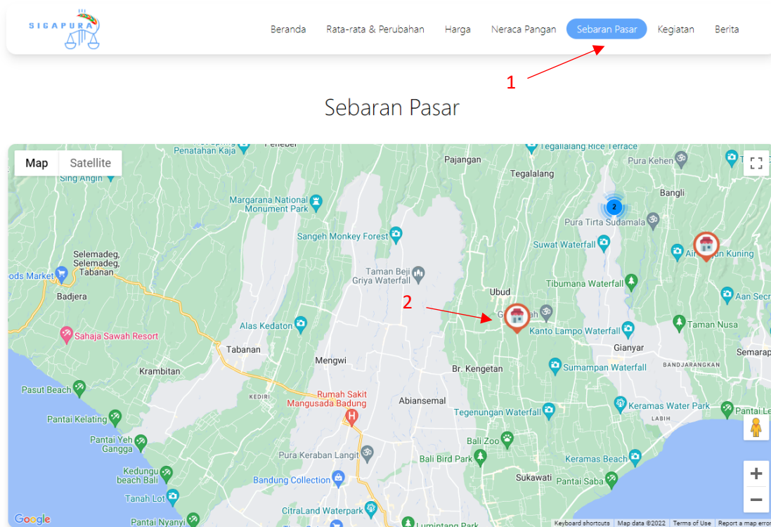
Gambar 8.7. Sebaran Pasar
